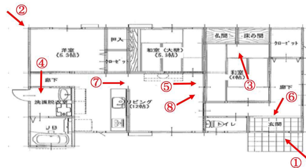
リフォーム後平面図
