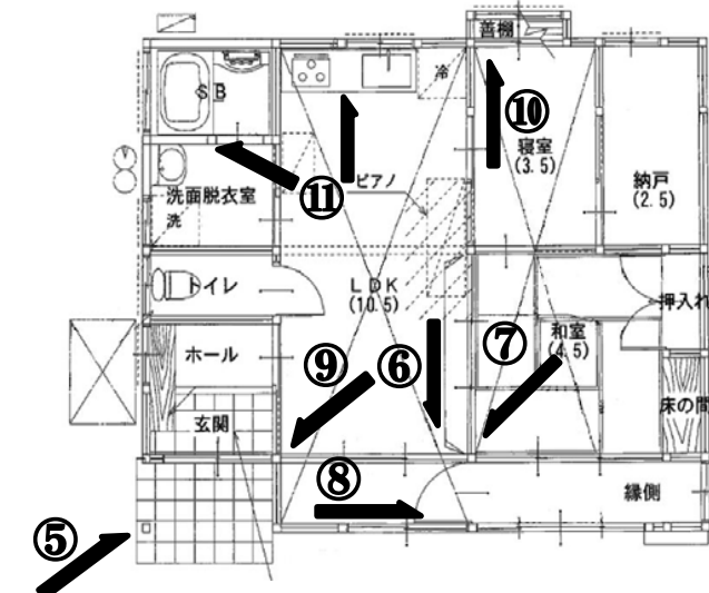
リフォーム後平面図
