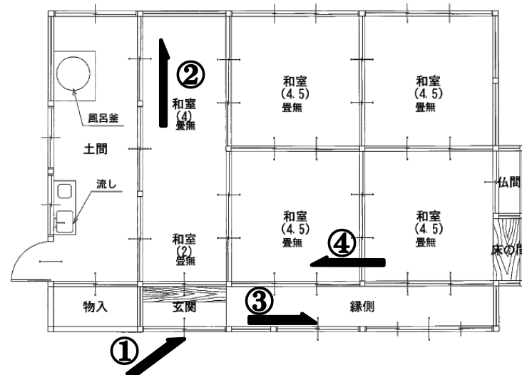
リフォーム前平面図
