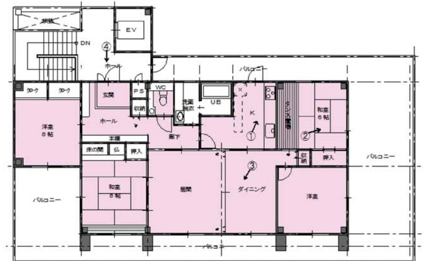
リフォーム前平面図
