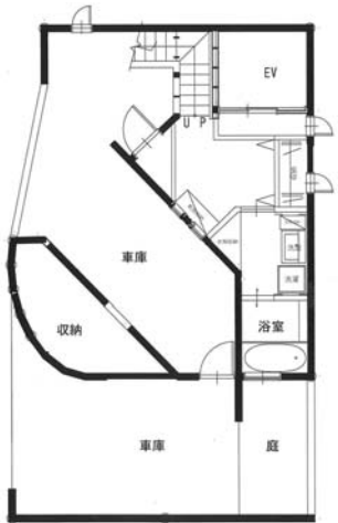
1 階平面図
