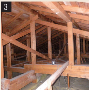
小屋裏
